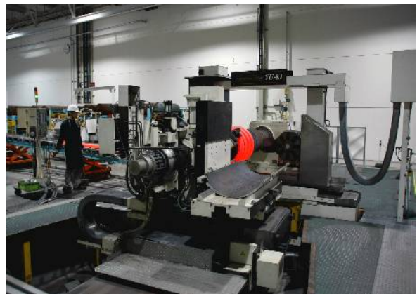
【ハイブリッド手づくり生産を象徴する大型バネ製造機「YU-KI」】
